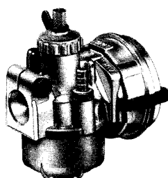
Schiebervergaser SRH ø 14
