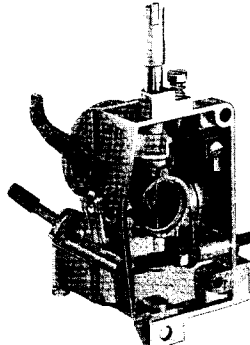
Drosselklappenvergaser 92 ø 16
