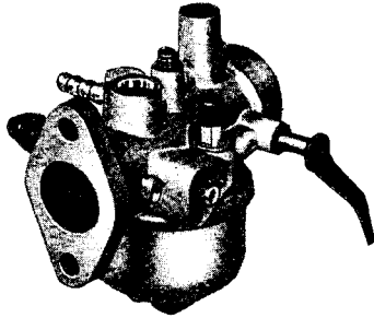
Drosselklappenvergaser DRA ø 14-18
