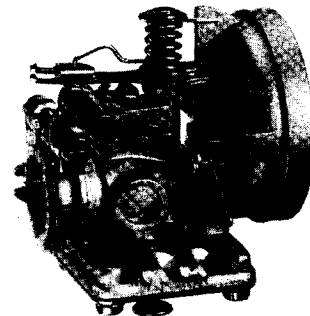
Membranvergaser 33-3 ø 10-15
