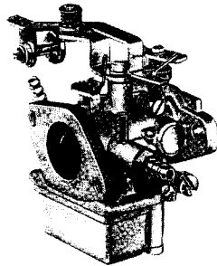
Drosselklappenvergaser 86 ø 12-14
